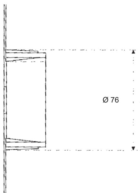
Coupe A-A
